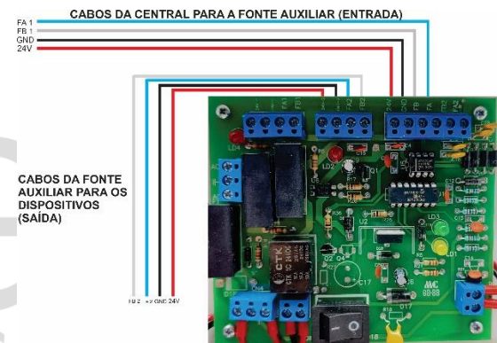
PLACA DA FONTE AUXILIAR SMAY 120E
